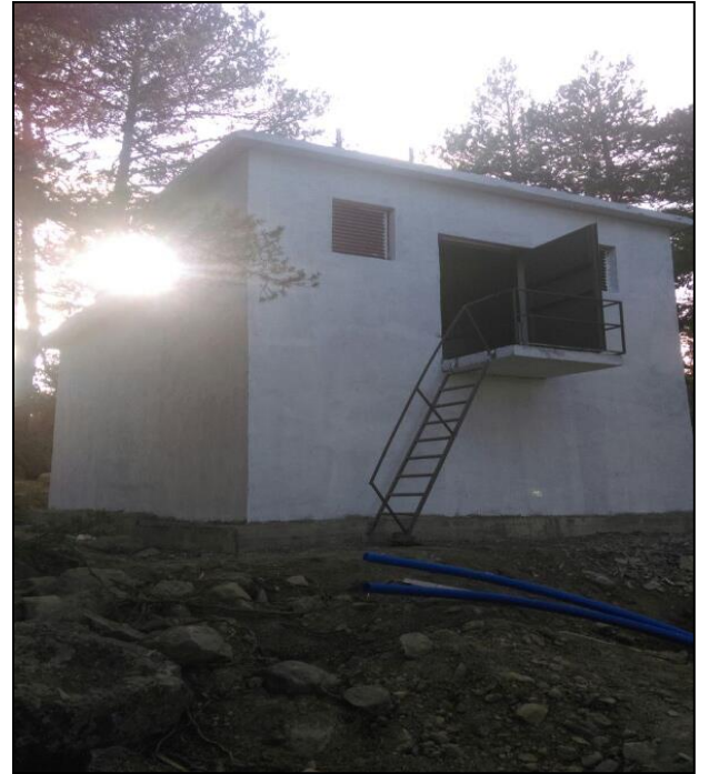
Seben Göleti Adro- Park 1 adet 50 m3 G.Depo yapımı görünümü
